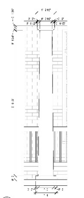
4 PORTICO COLUMN - STUDY SCALE: 3/8" = 1'-0"
